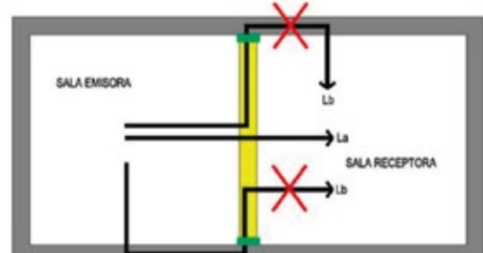
APLICACIÓN DE BANDA PARA EVITAR LA TRANSMISIÓN DE SONIDOS POR EL CONTORNO Banda de Estanqueidad Acústica knauf
