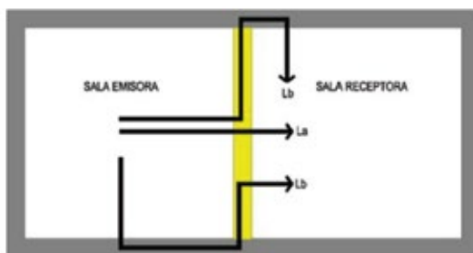
SITUACIÓN EN TERRENO TRANSMISIÓN DE SONIDOS POR CONTORNO
